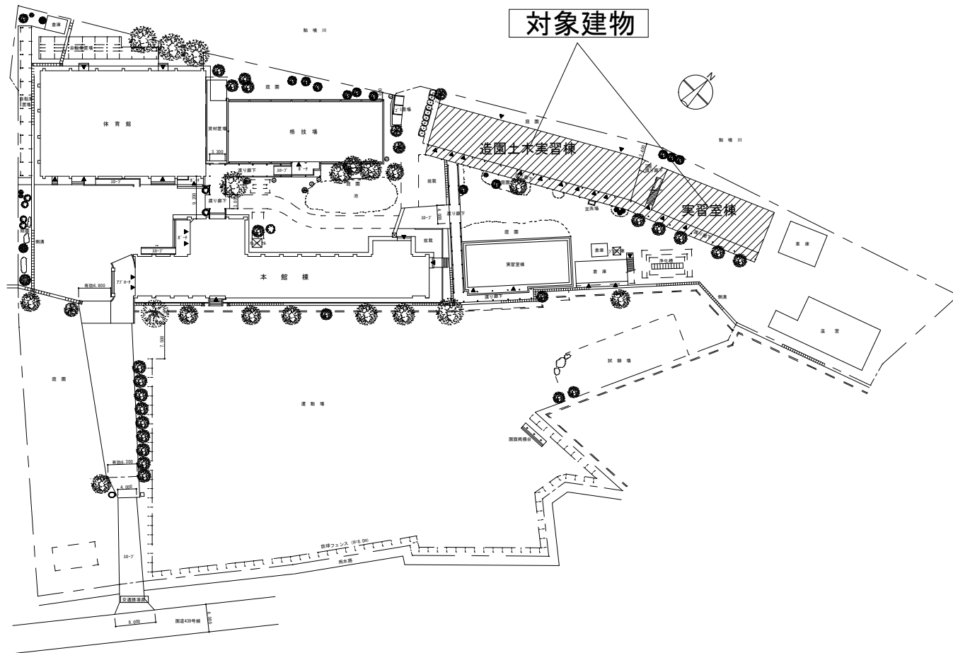
全体配置図 1:600
